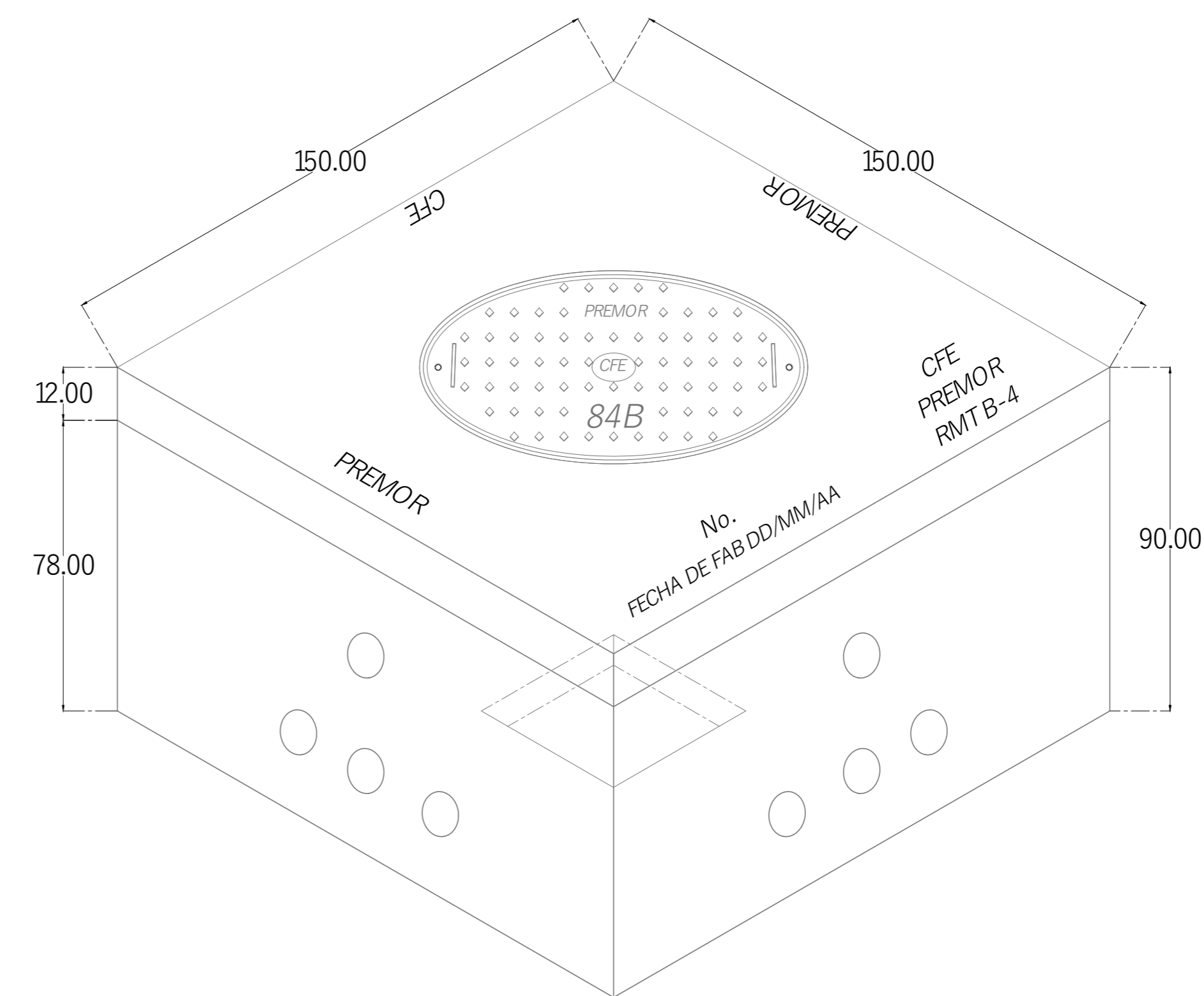
ISOMETRICO
