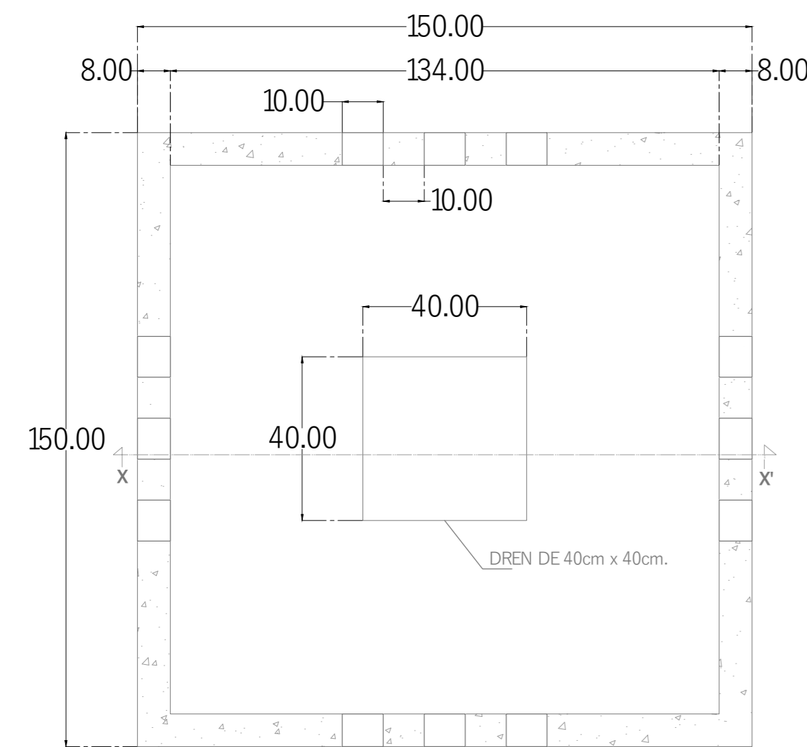
PLANTA
