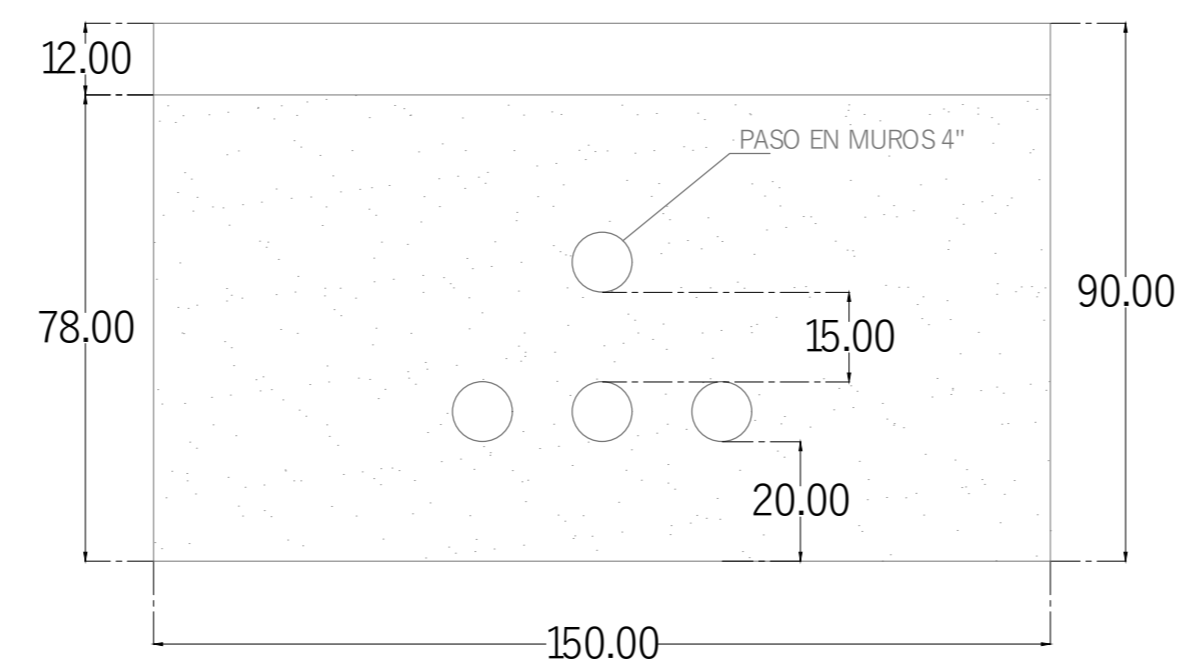
VISTA LATERAL
