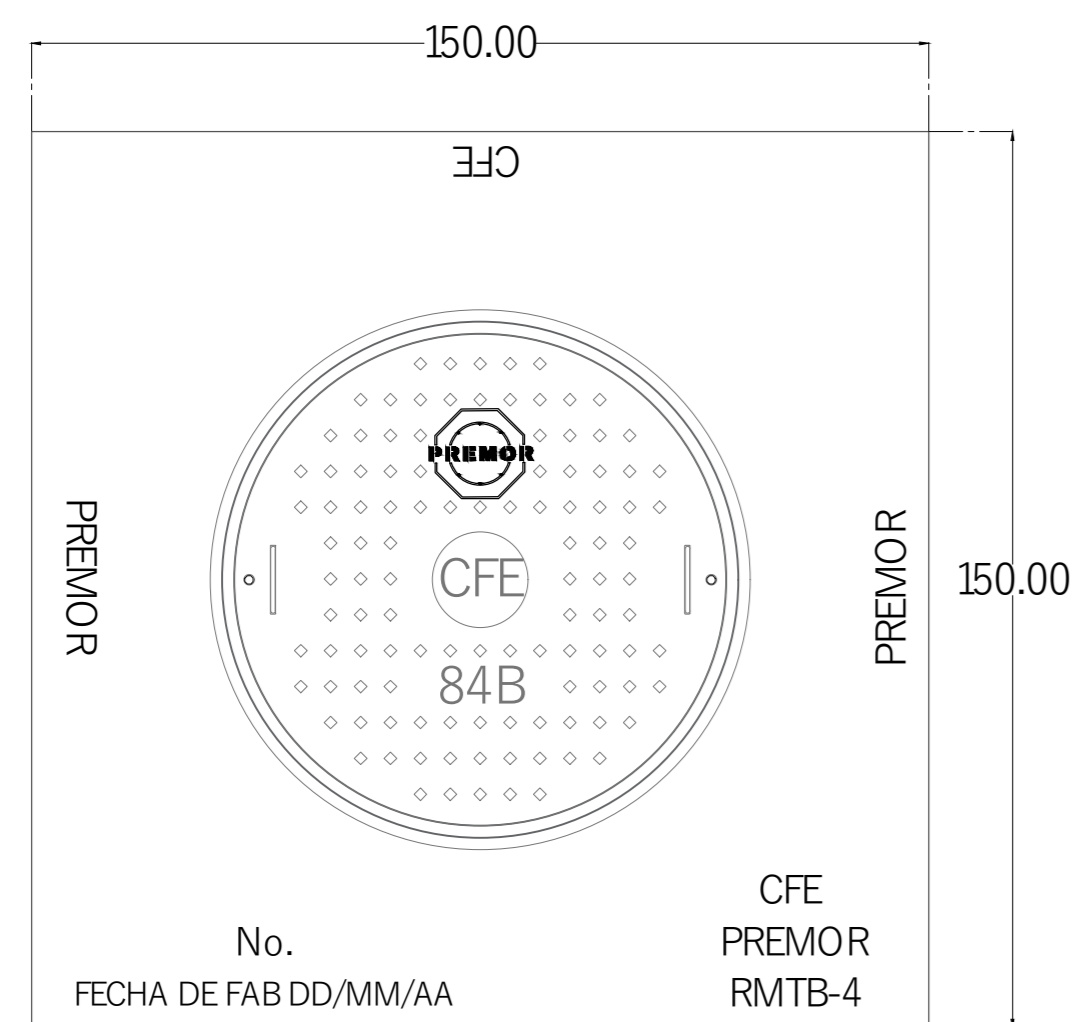
PLANTA TAPA
