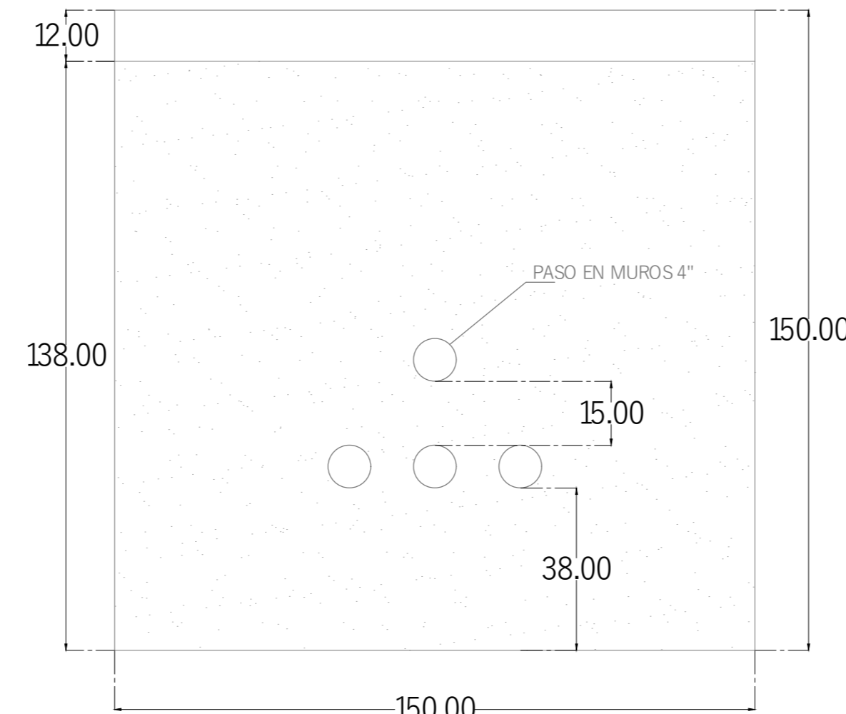
VISTA LATERAL
