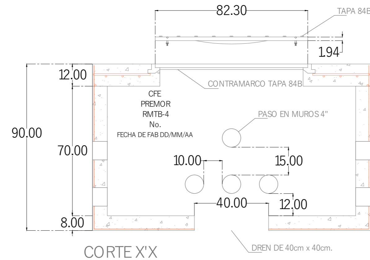
CORTE X'X
