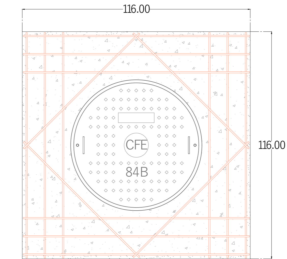
ARMADO DE LOSA
