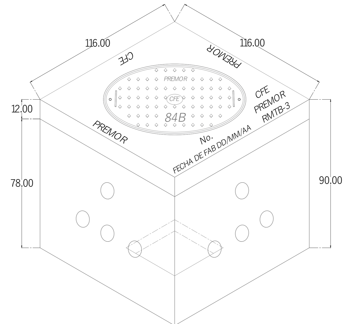
ISOMETRICO
