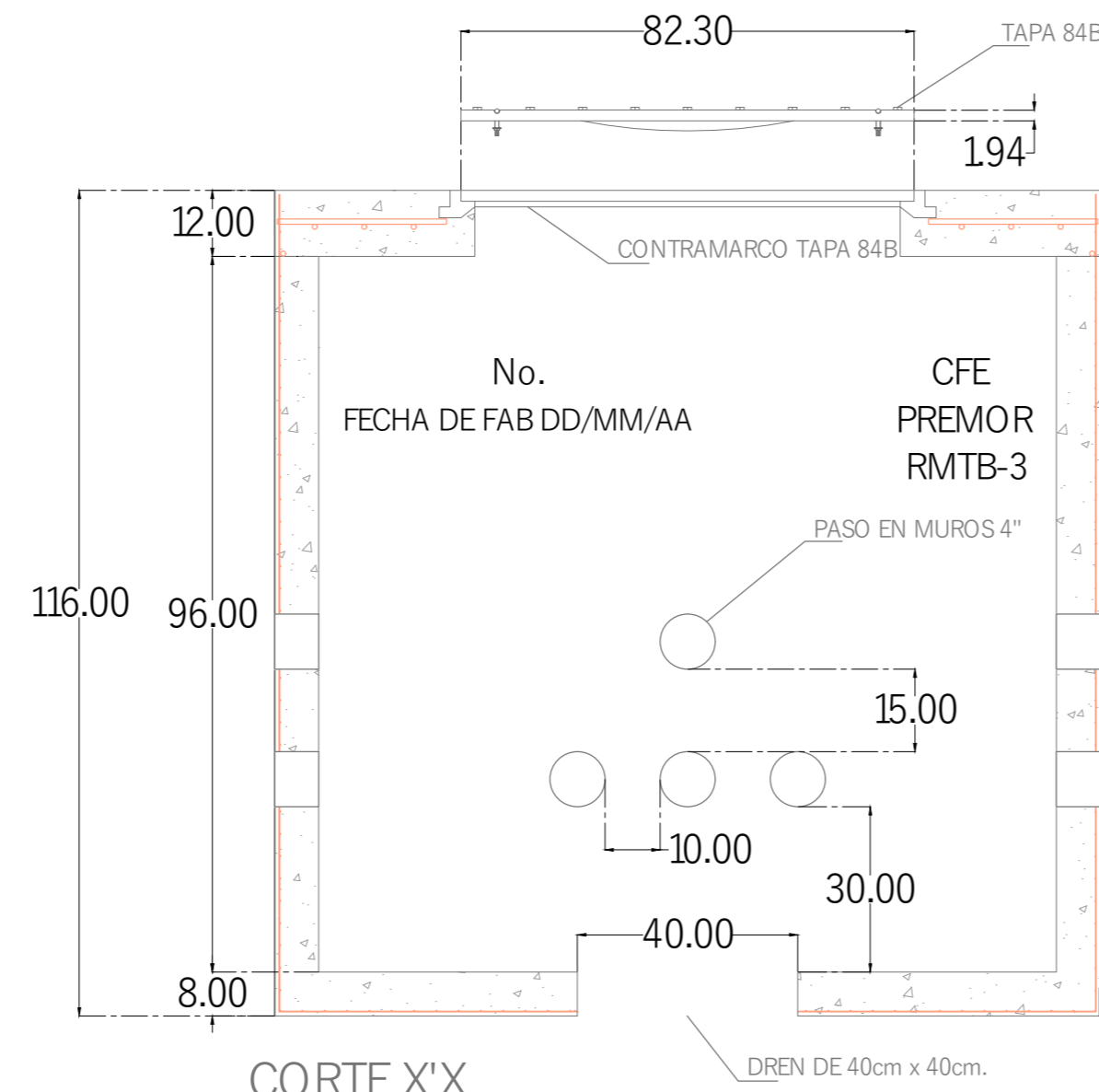
CORTE X'X
