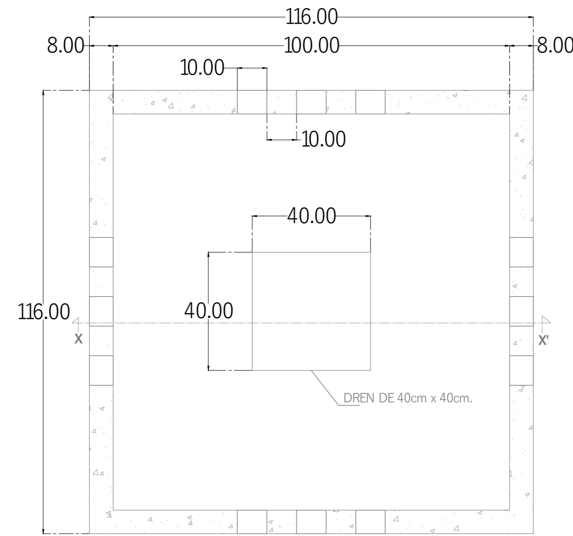
PLANTA
