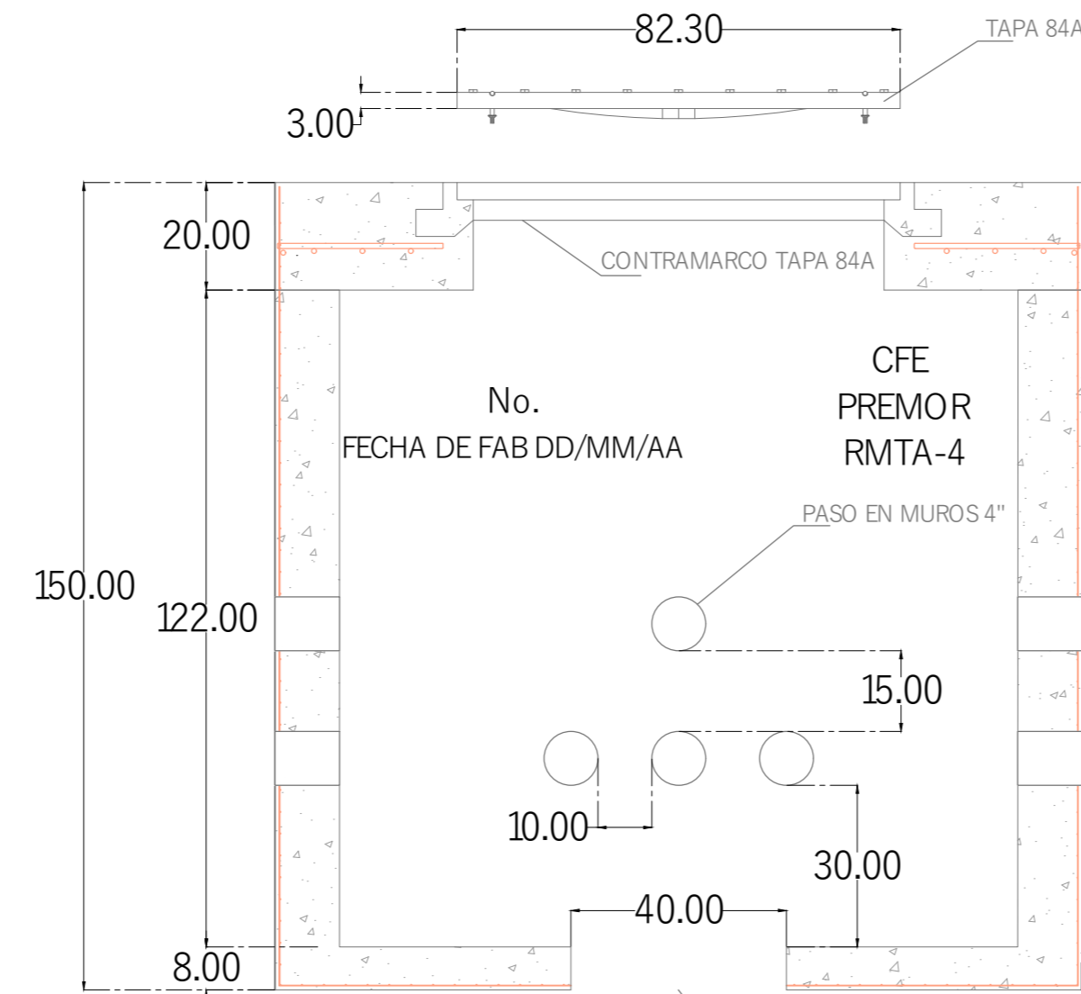
CORTE X'X
