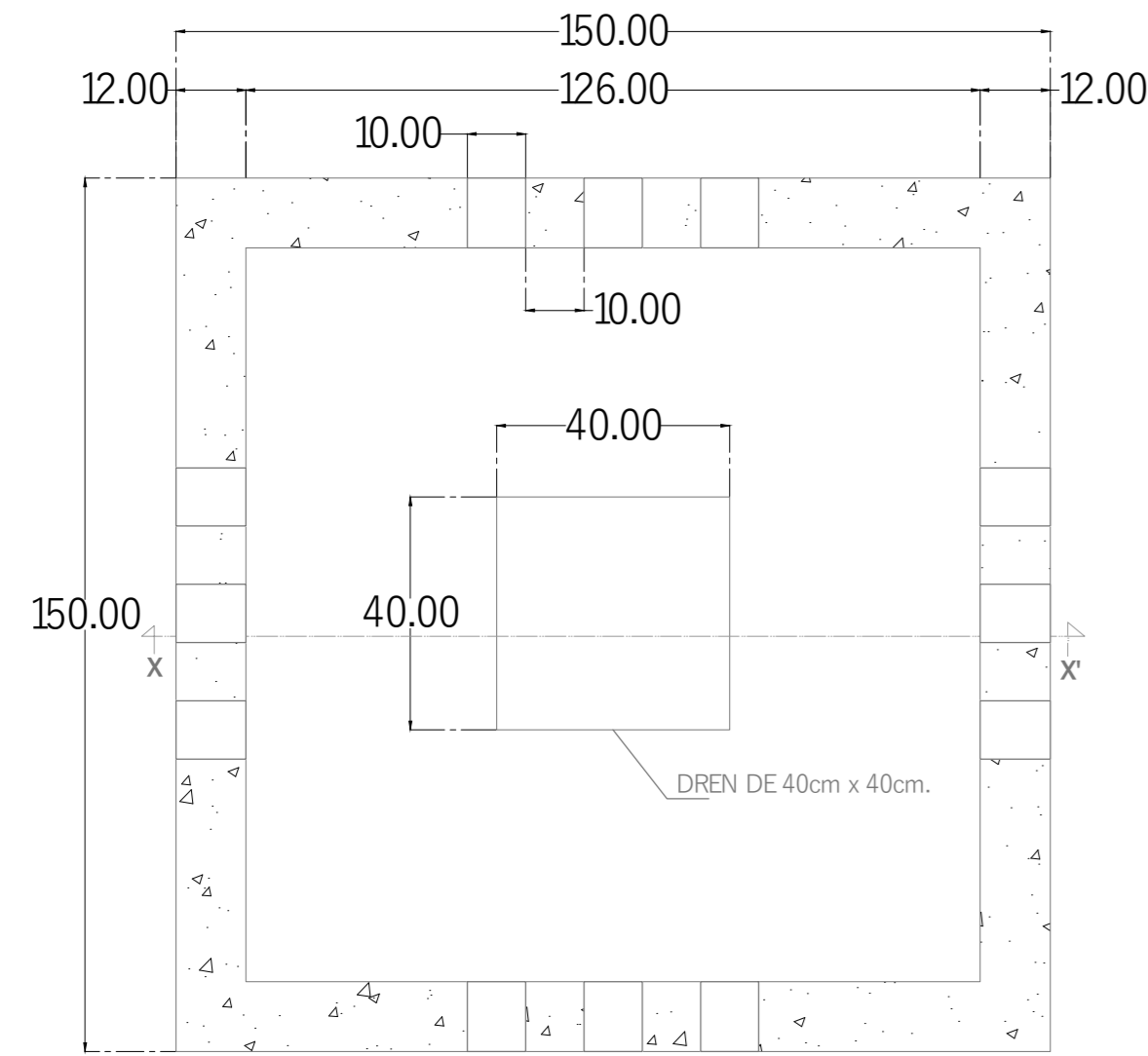
PLANTA
